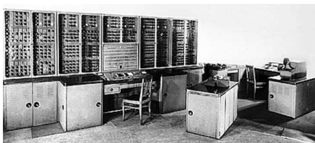
Част от блоковете на електронно-изчислителната машина „Урал-1“
